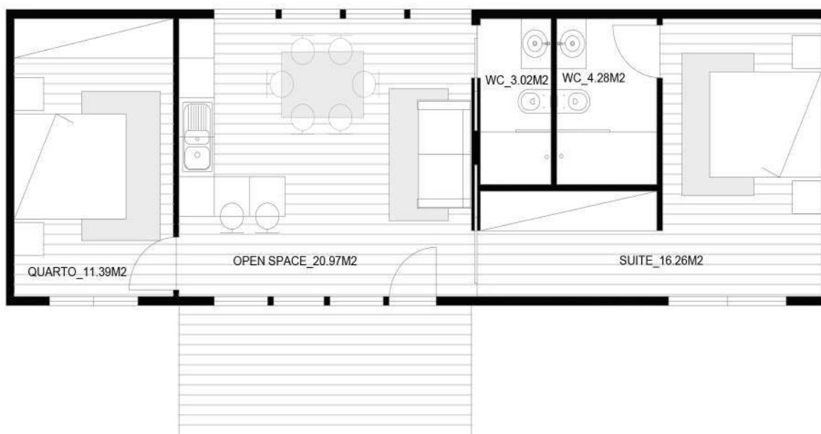
PLANTA PISO 0_63.00m2
